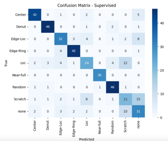
<그림 9> 지도 학습 Confusion Matrix
